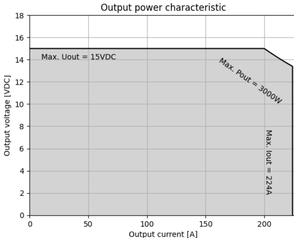
Abbildung 9.1: Ausgangsleistung DVCH3003-400-12
