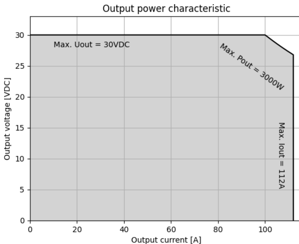
Abbildung 9.2: Ausgangsleistung DVCH3003-400-24
