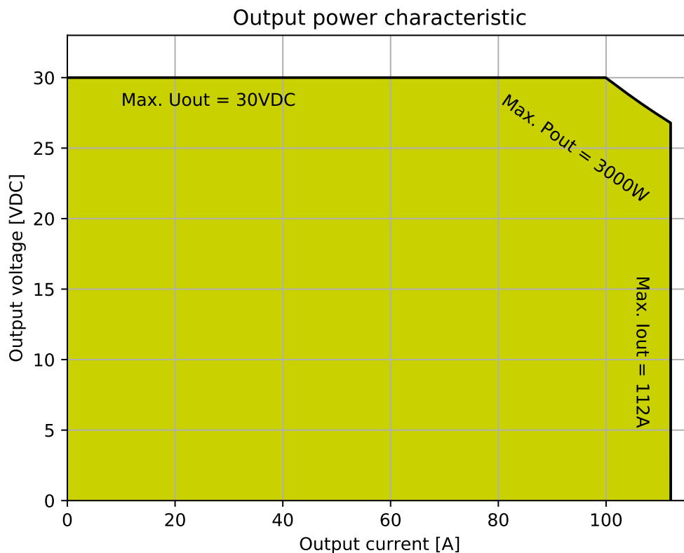
Abbildung 9.2: Ausgangsleistung DVCH3003-700-24
