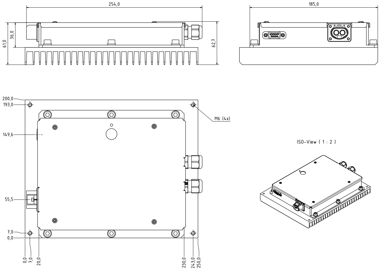
Abbildung 9.1: Dimensions
