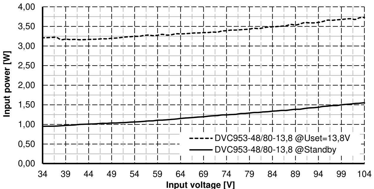
Abbildung 10.2: No-load input power
